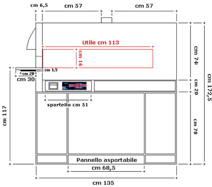
Prospetto Laterale
