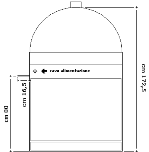
Prospetto Posteriore
