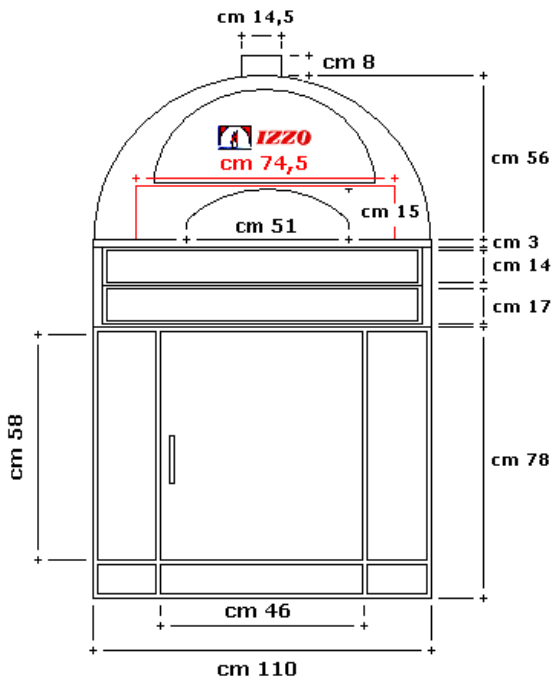
Prospetto Frontale
