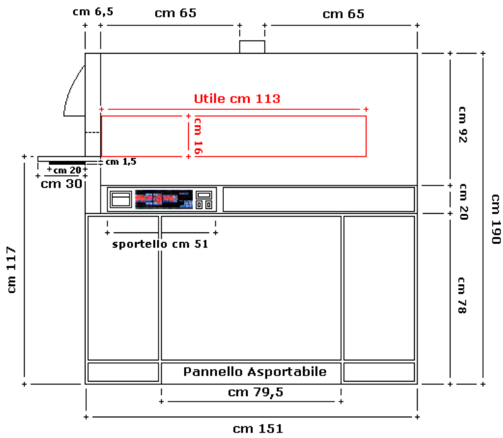
Prospetto Laterale
