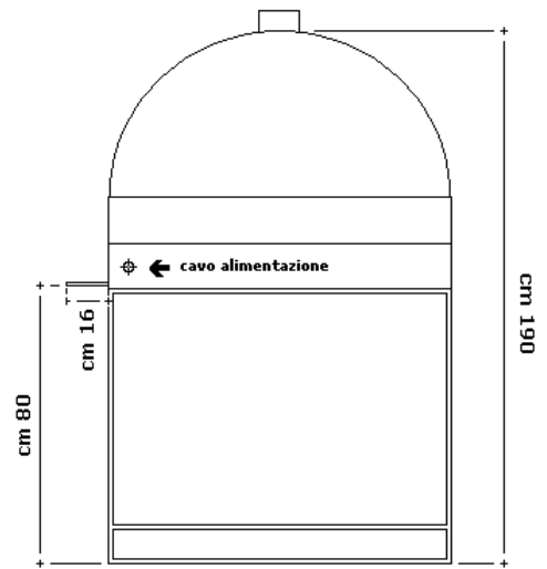
Prospetto Posteriore
