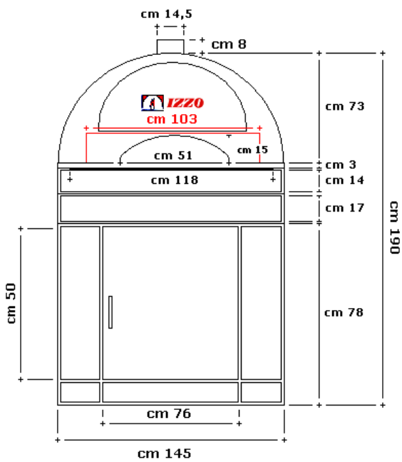
Prospetto Frontale
