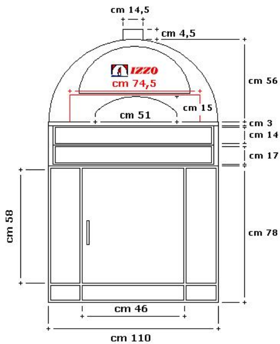
Prospetto Frontale
